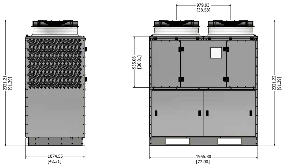
VISTA LATERAL
