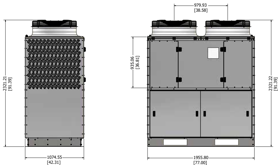
VISTA LATERAL
